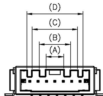
07~12 Pin
